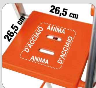
Pedana a getto di resina con anima di rinforzo d'acciaio.
